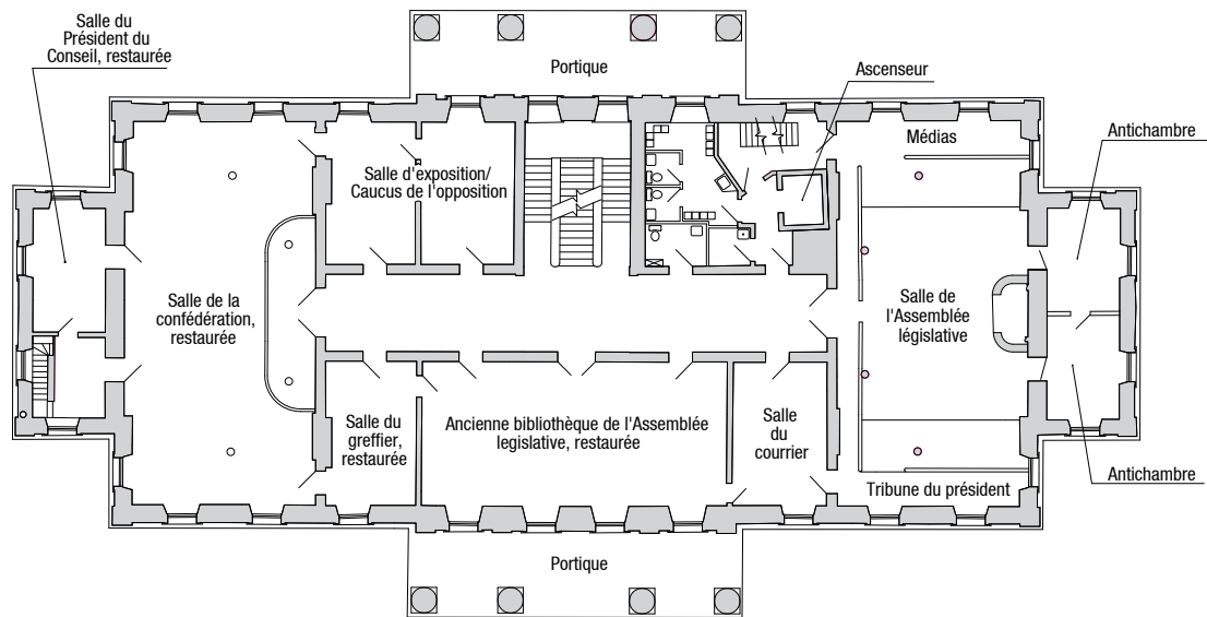
1 er étage
